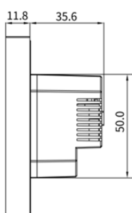
② ВИД СПРАВА
